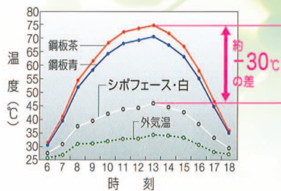
屋根表面温度シミュレーション
