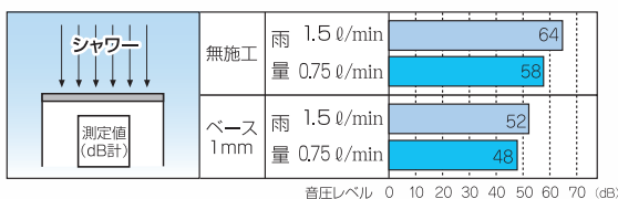
雨音消音性能(シャワーテストはベース1mmで測定)
