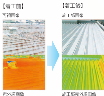
屋根表面温度シミュレーション
